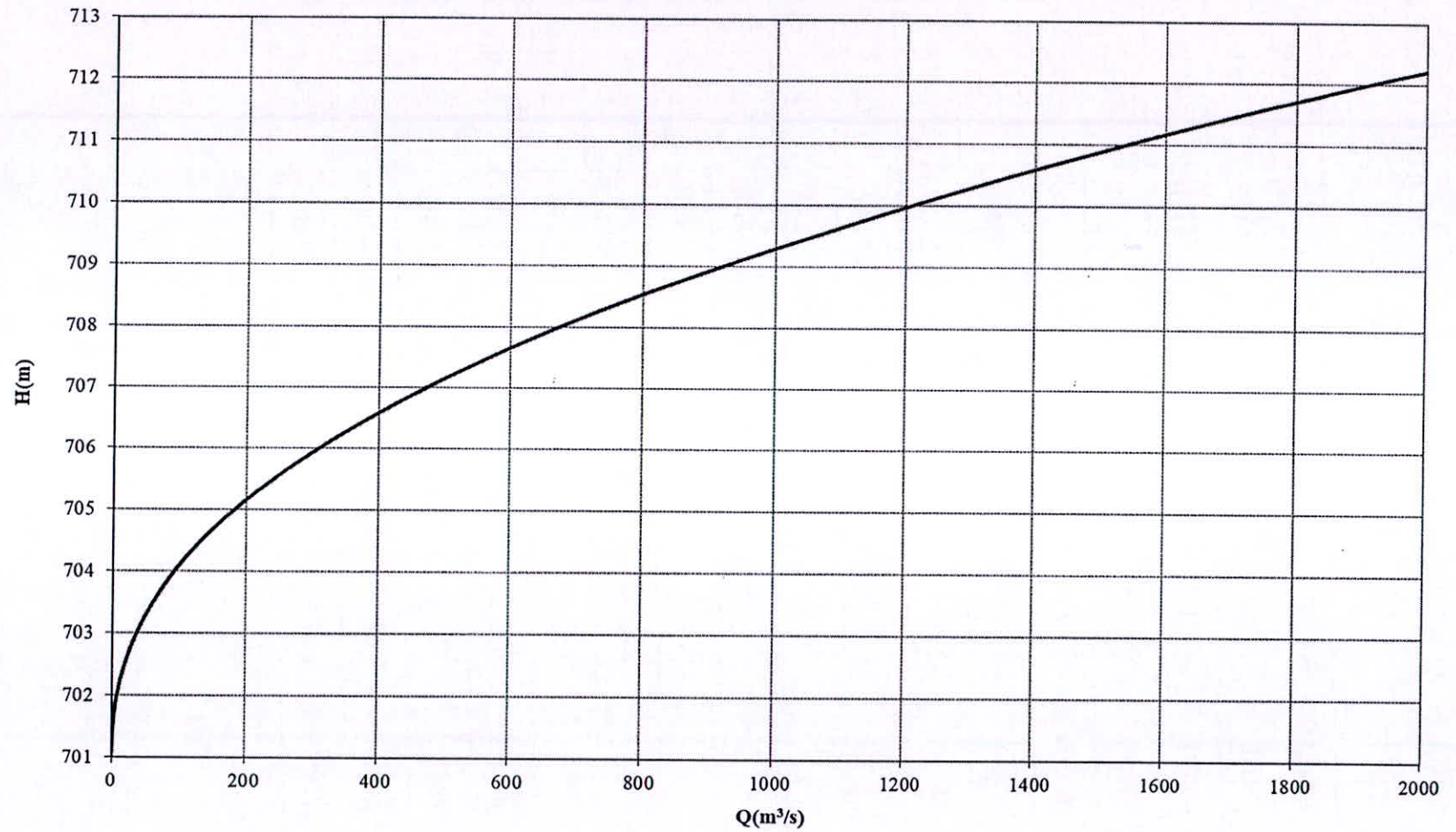
QUAN HỆ Q=f(H) HẠ LƯU TUYẾN ĐẬP
